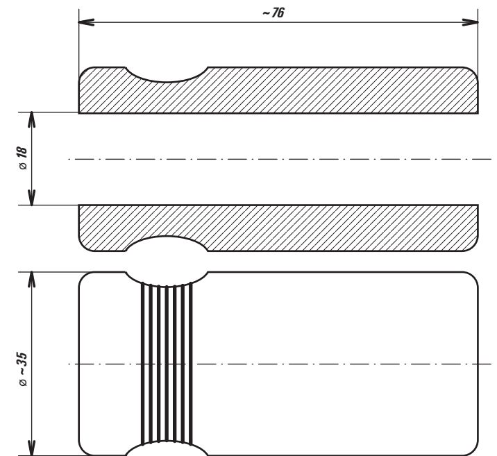
Aufnahmeteil für Bordunpfeife
