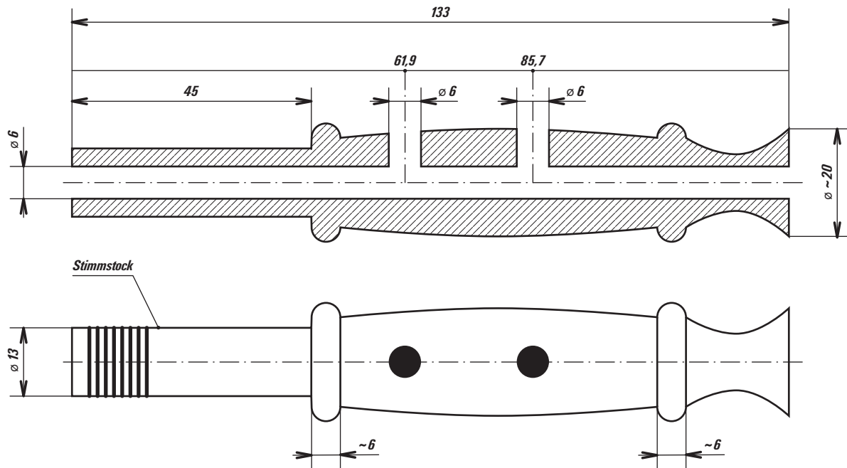
Das obere Teil der Bordunpfeife
