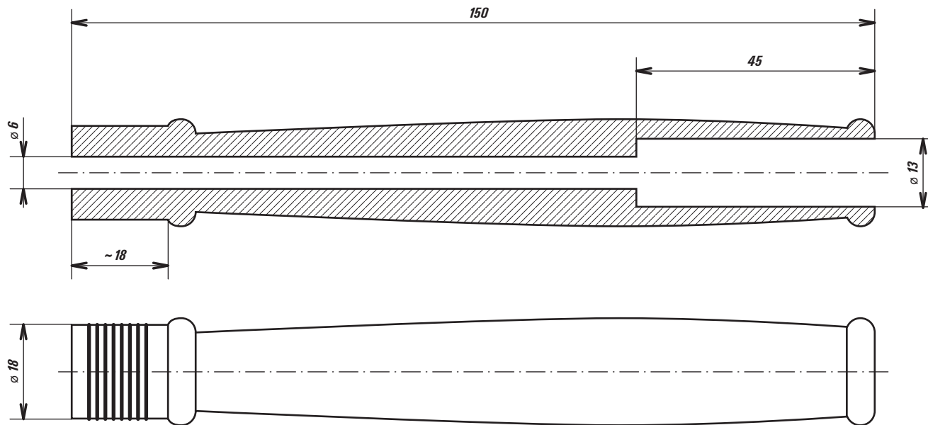
Das untere Teil der Bordunpfeife
