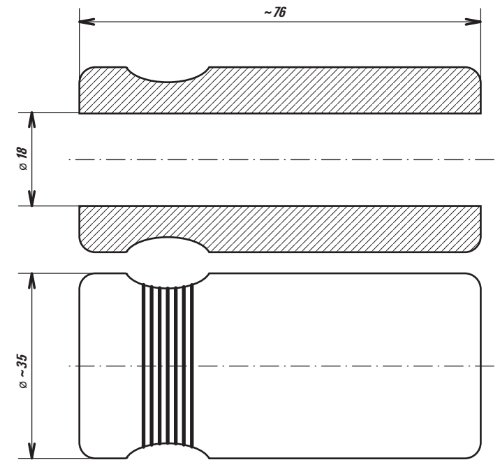
Aufnahmeteil für Melodiepfeife
